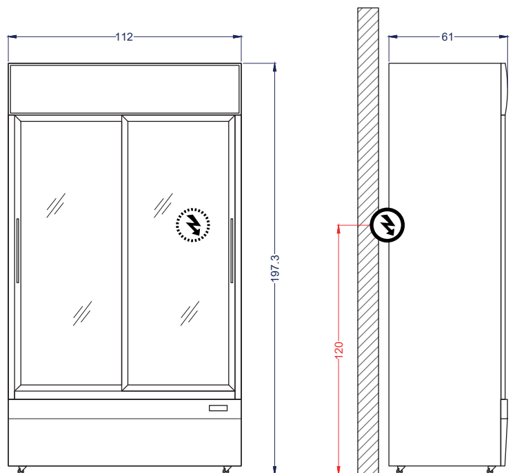
Vista Elevación
